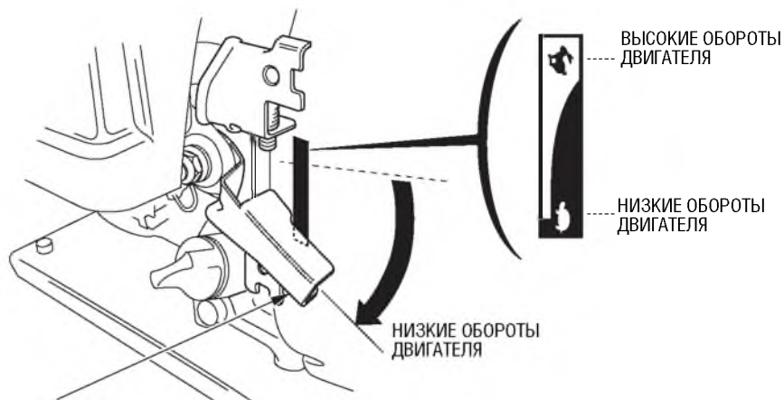
РЫЧАГ УПРАВЛЕНИЯ ДРОССЕЛЬНОЙ ЗАСЛОНКОЙ
