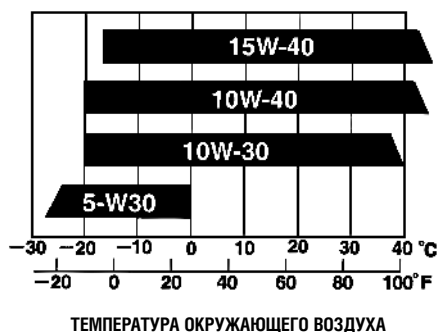
Температурный диапазон применяемости масел
