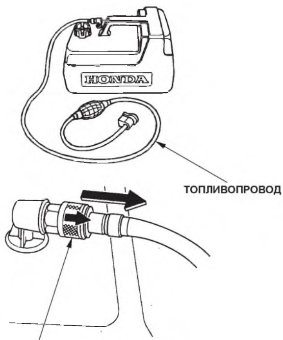
ШТУЦЕР ДЛЯ ПРИСОЕДИНЕНИЯ ТОПЛИВОПРОВОДА
