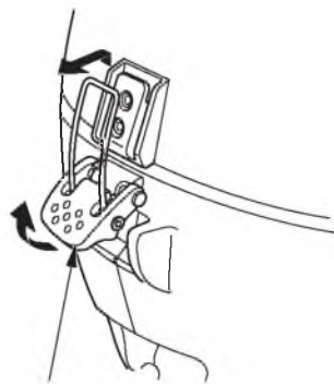
ЗАМОК ВЕРХНЕГО КОЖУХА ДВИГАТЕЛЯ
