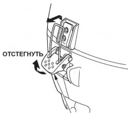
ЗАМОК ВЕРХНЕГО КОЖУХА ДВИГАТЕЛЯ
