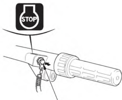
ВЫКЛЮЧАТЕЛЬ ДВИГАТЕЛЯ
