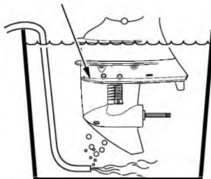
АНТИКАВИТАЦИОННАЯ ПЛИТА
