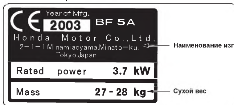
СЕРТИФИКАЦИОННАЯ ТАБЛИЧКА
