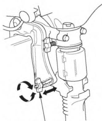
РЕГУЛИРОВОЧНЫЙ БОЛТ И ГАЙКА-БАРАШЕК
