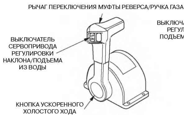
ПУЛЬТ ДЛЯ УСТАНОВКИ СВЕРХУ (модификация R3) (ДЛЯ ОДНОМОТОРНОГО СУДНА)
